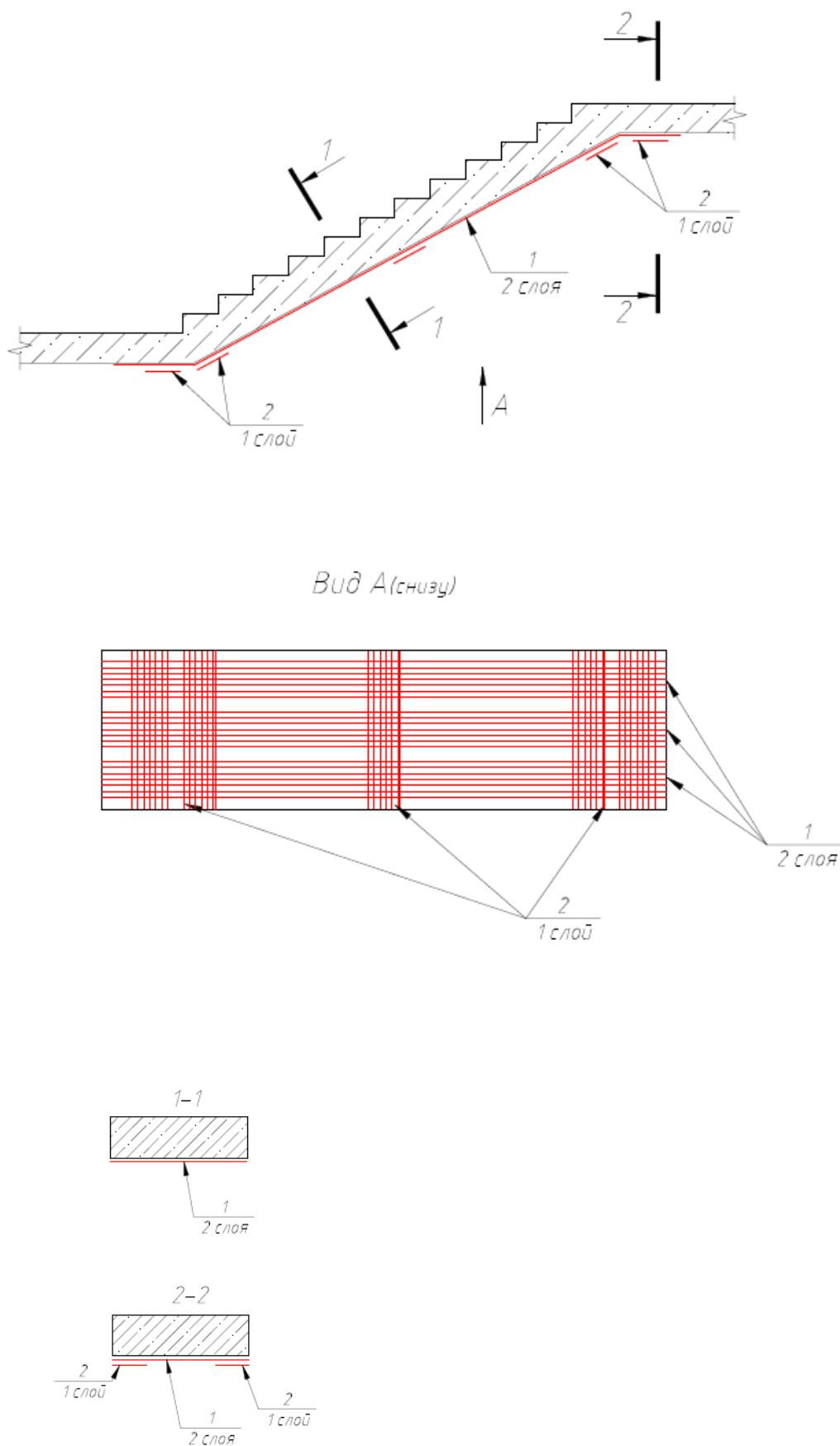
Рисунок 5.85 Пример усиления лестничного марша углеродными лентами CarbonWrap® Tape
