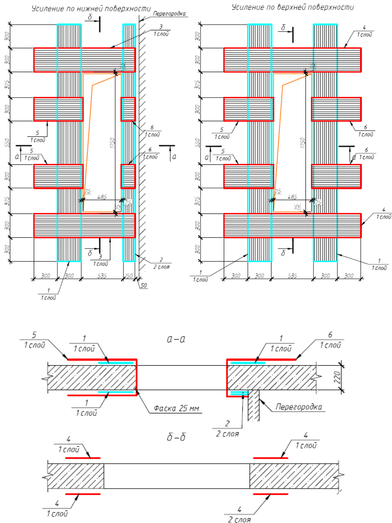
Рисунок 5.91 Пример устройства отверстия в монолитном перекрытии
